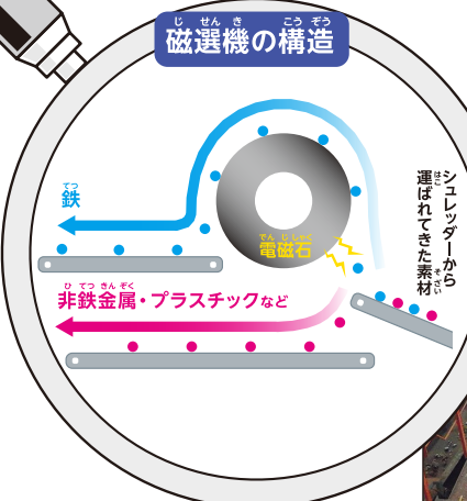
金属資源等の素材ごとの分別は、まずそれぞれの性質を利用して機械で行われます
